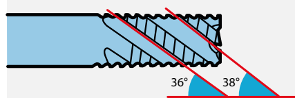
HS 100 U (Typ NF)
