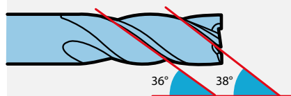
TF 100 INOX (Typ N)
